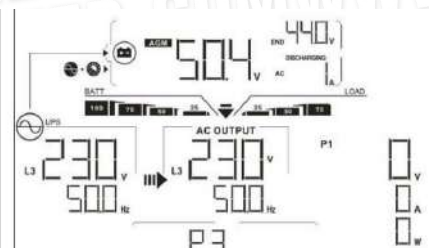
Affichage LCD dans l'unité L3-phase
