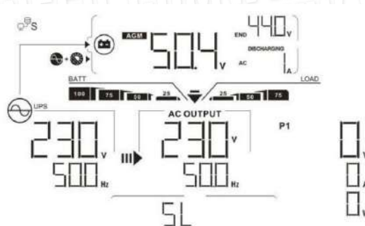
Affichage LCD dans l'unité esclave
